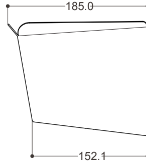
Vista Laterale
