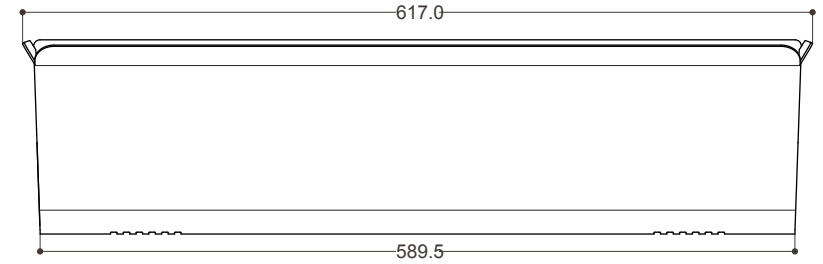
Vista Frontale
